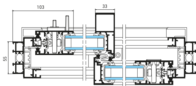
2 vantaux - 2 rails
