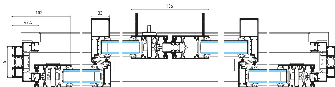
4 vantaux - 2 rails
