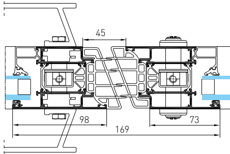
Nœud central porte 2 vantaux
