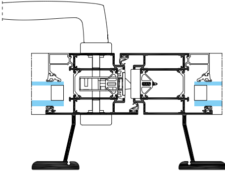
Noeud central porte grande hauteur 2 vantaux
