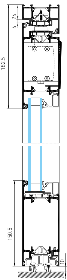
Coupe verticale complète sans seuil
