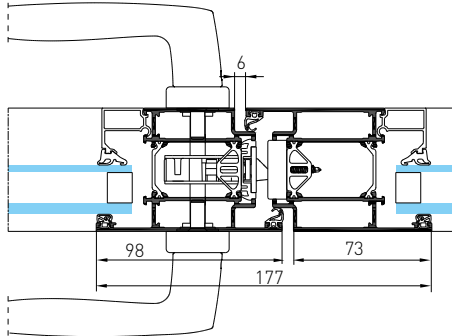
Nœud central porte 2 vantaux
