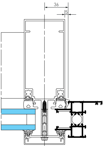
coupe ouverture extérieure
