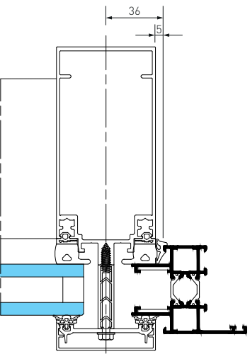
Coupe ouverture intérieure
