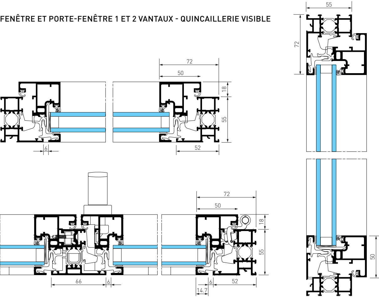
INTÉGRATION DANS FACADE MUR-RIDEAU (SPINAL)
