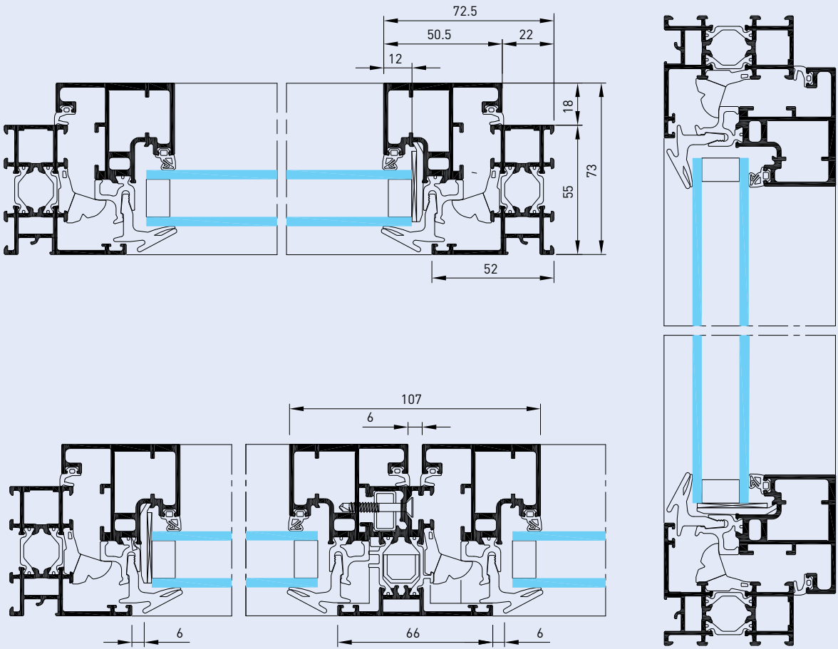
FENÊTRE ET PORTE-FENÊTRE 1 ET 2 VANTAUX - QUINCAILLERIE CACHÉE
