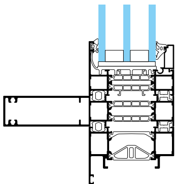
SOLEAL Next 75 Ensemble composé avec montant renforcé et intégration porte
