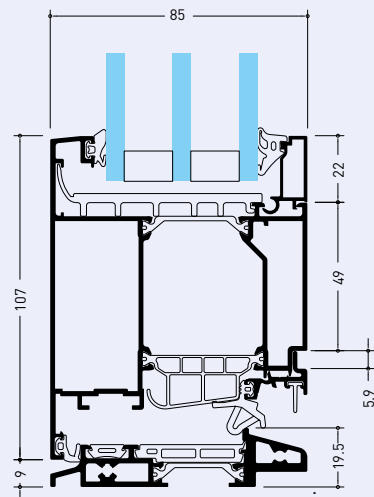
Porte résidentielle, Ouverture extérieure, Seuil PMR
