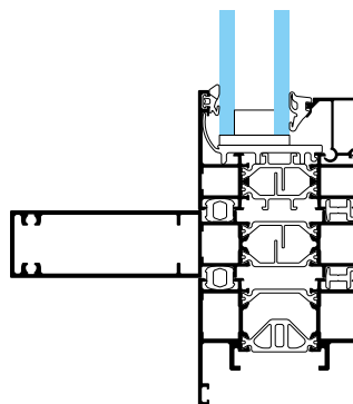
SOLEAL Next 65 Ensemble composé avec montant renforcé et intégration porte
