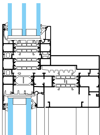
SOLEAL Next 75 Ensemble composé avec le couissant à frappe TIGAL
