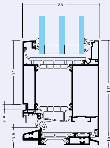
Porte résidentielle, Ouverture intérieure, Seuil PMR
