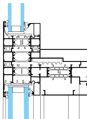
SOLEAL Next 65 Ensemble composé avec le couissant à frappe TIGAL
