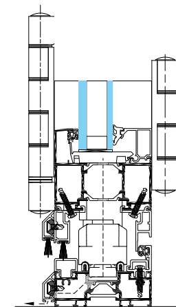
Drainage caché en option dans toutes les applications
